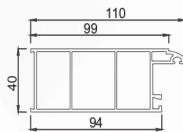
80 Door Sash PM80-2 (1.076 kg/m) 4 pieces/bag
