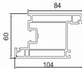
60 Inward Door Sash PM60-1 (1.524 kg/m) 4 pieces/bag
